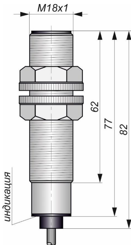
Габаритный чертеж
